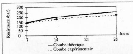
Figure 2 : Variation de la résistance du béton en fonction de l'âge.
