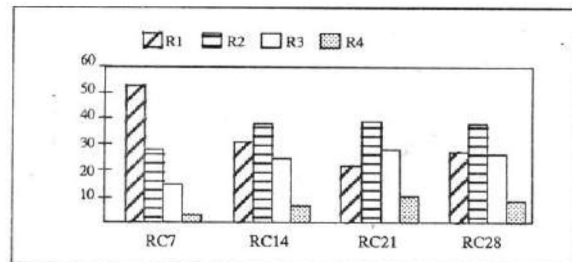
Figure 1 : Distribution des résistances dans les intervalles R1, R2, R3, et R4.
