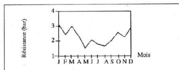
Figure 4a : Distribution mensuelle des résistances à 28 jours de classe I (R1).
